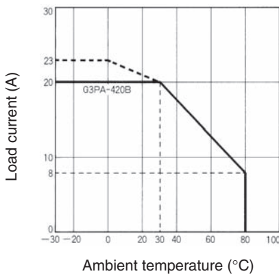
G3PA-420B-VD, G3PA-420B-VD-2
